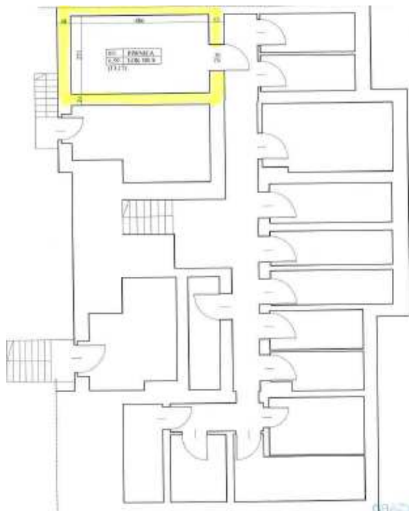
Rzut piwnicy
